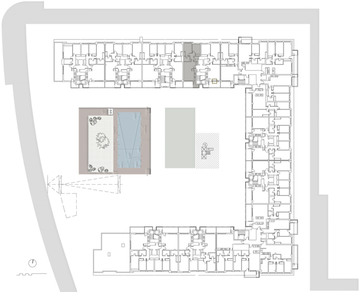
PORTAL 4 PLANTA 1-4 PISO A
